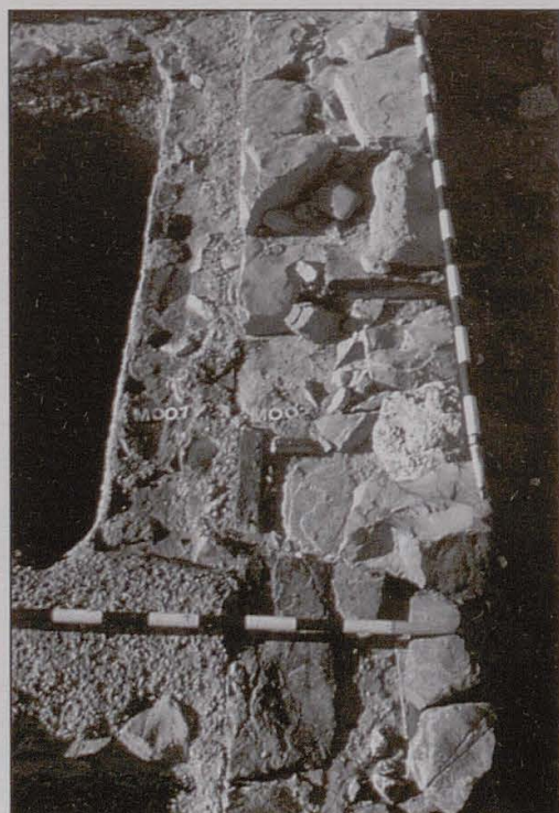
Figura 12 B. Detalles constructivos del Conjunto Industrial I. Detalle de la zona de unión de la pila nororiental del C.I. con el muro perimetral este del citado conjunto, con la indicación del recrecimiento murario hacia el interior de la cubeta tras la reforma.
