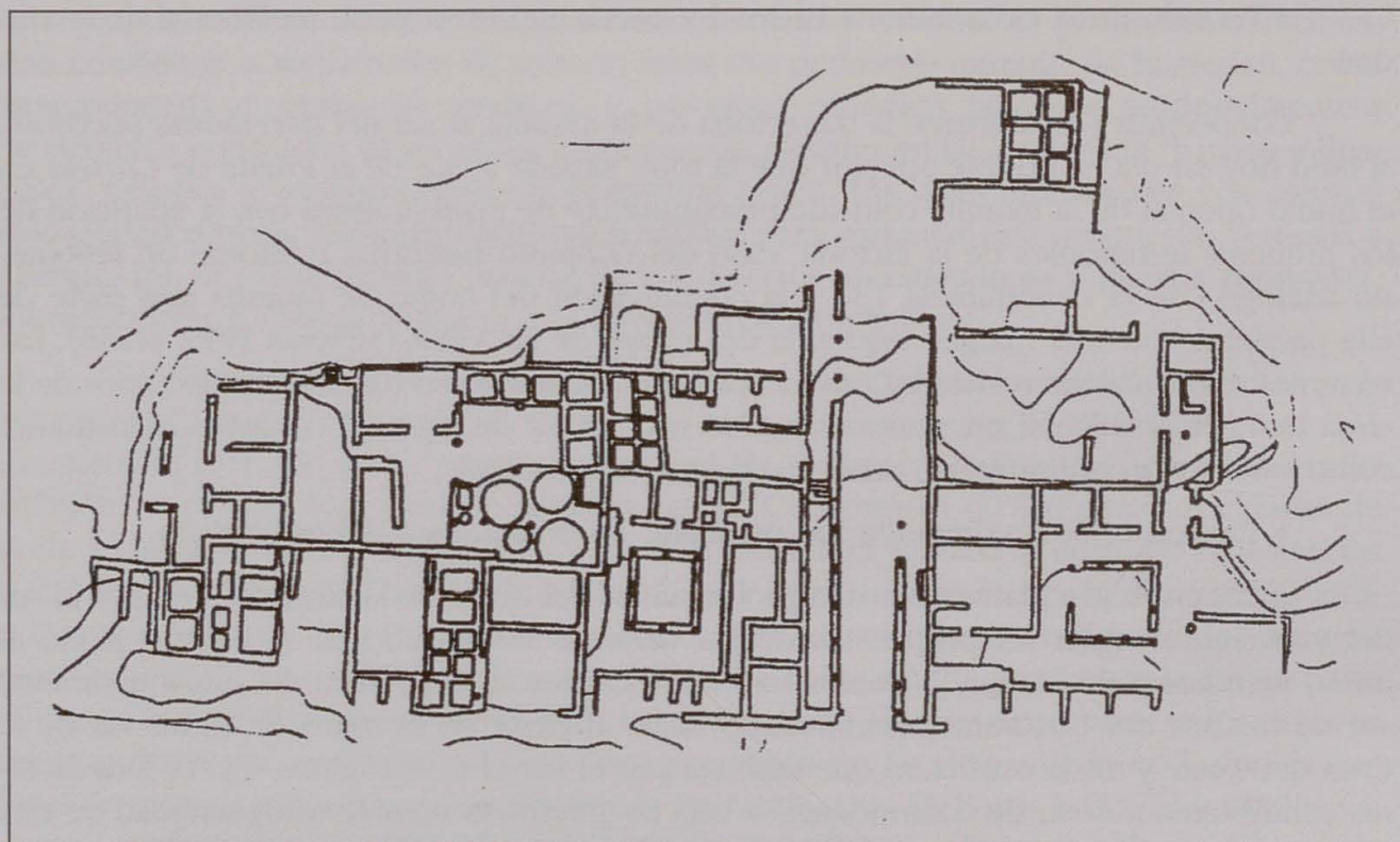
Figura 5. Planimetría de la factoría de Baelo Claudia , procedente de la cartografía informatizada del Conjunto Arqueológico (Consejería de Cultura de la Junta de Andalucía)
