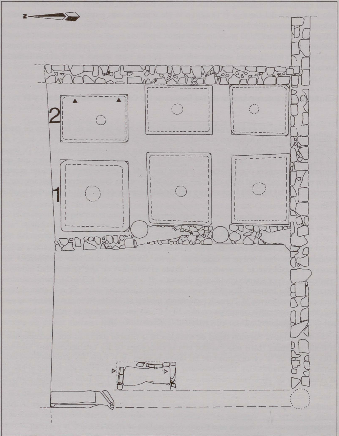
Figura 10. Planta general del Conjunto Industrial I, en la Zona Oriental del Barrio Industrial (Dibujo L. Aguilera)
