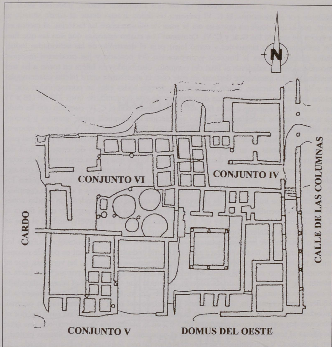
Figura 7. Zona central de la factoría con la indicación de los Conjuntos Industriales IV, V y VI, así como la Casa del Oeste
