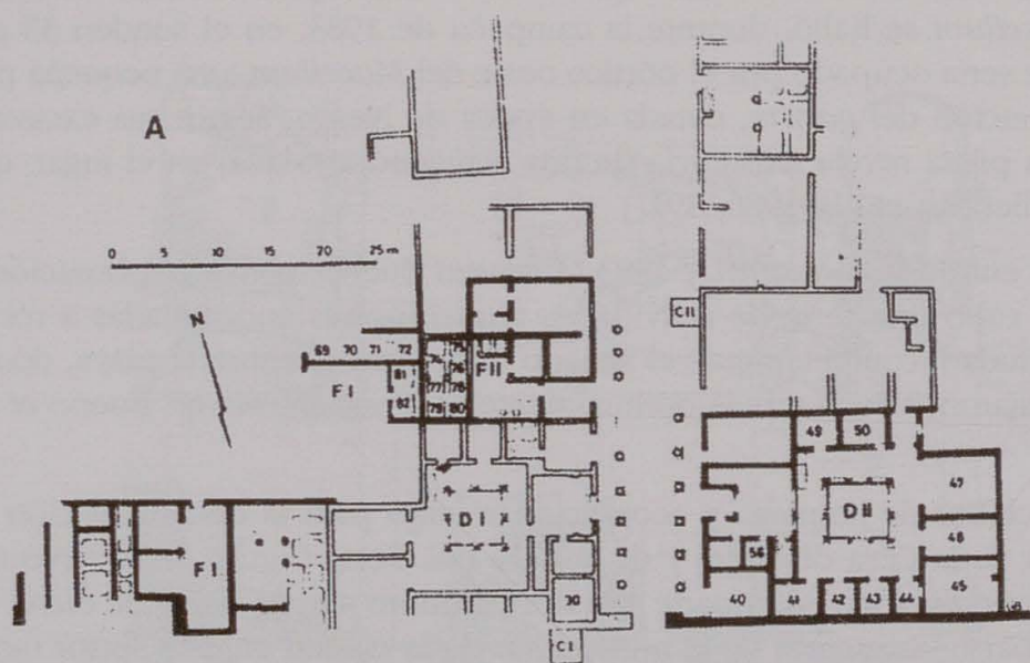
Planimetría de la factoría según Martín Bueno (1984)
