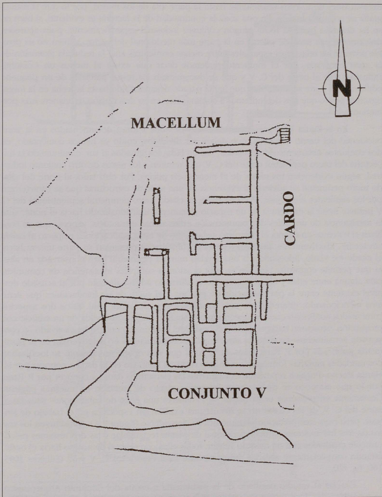
Figura 8. Zona occidental de la factoría con indicación del posible macellum y de la zona parcial de otro conjunto industrial
