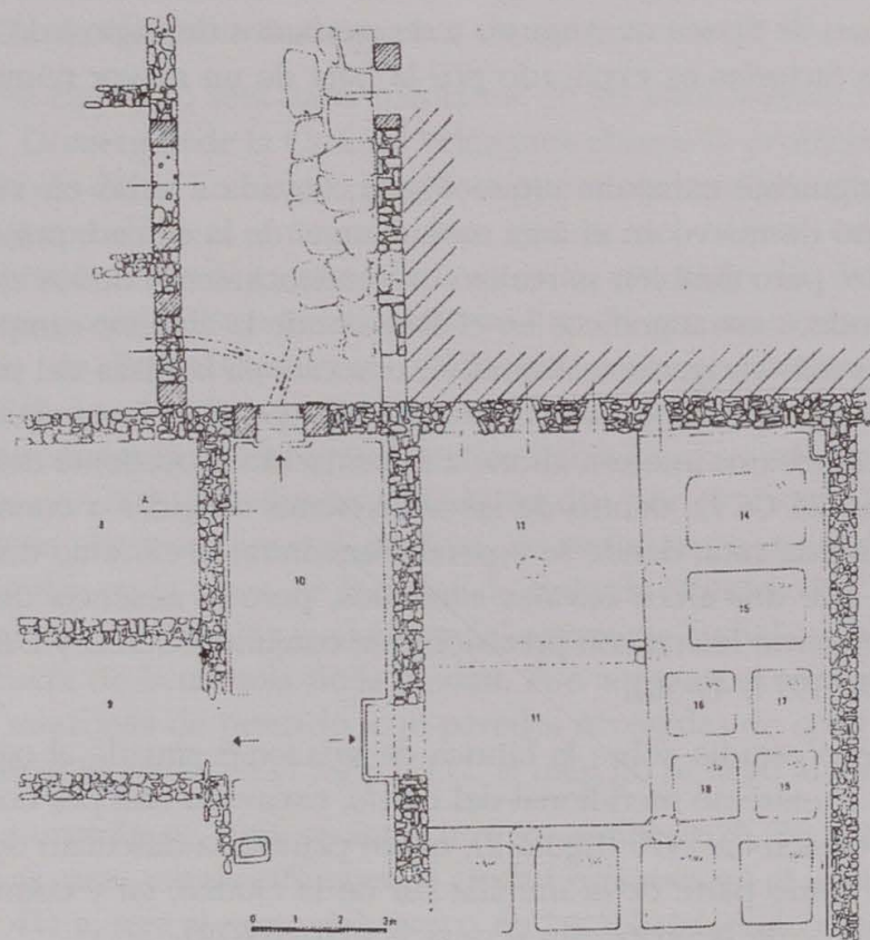
Planta de uno de los conjuntos industriales según Ponsich (MCV XII)
