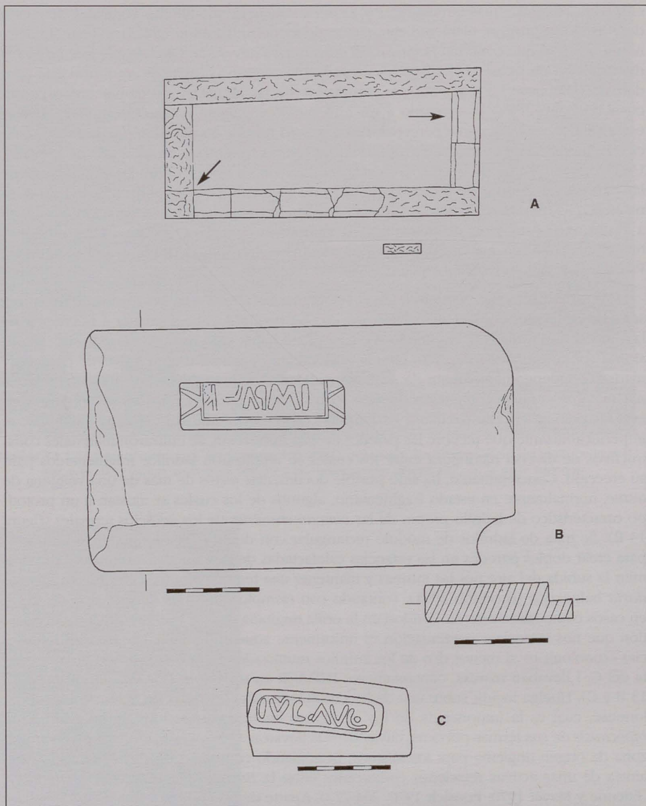
Figura 13. Detalle de los materiales constructivos de la pila cuadrangular del C.I. con los sellos latericios (dibujo de L. Lorenzo). A. Planta de la pila rectangular, con indicación de los ladrillos reutilizados. B. Ladrillo de termas con la marca IMP ACR (retro) in tabula ansata . C. Detalle del ladrillo con la marca IVL.AVG en cartella rectangular.
