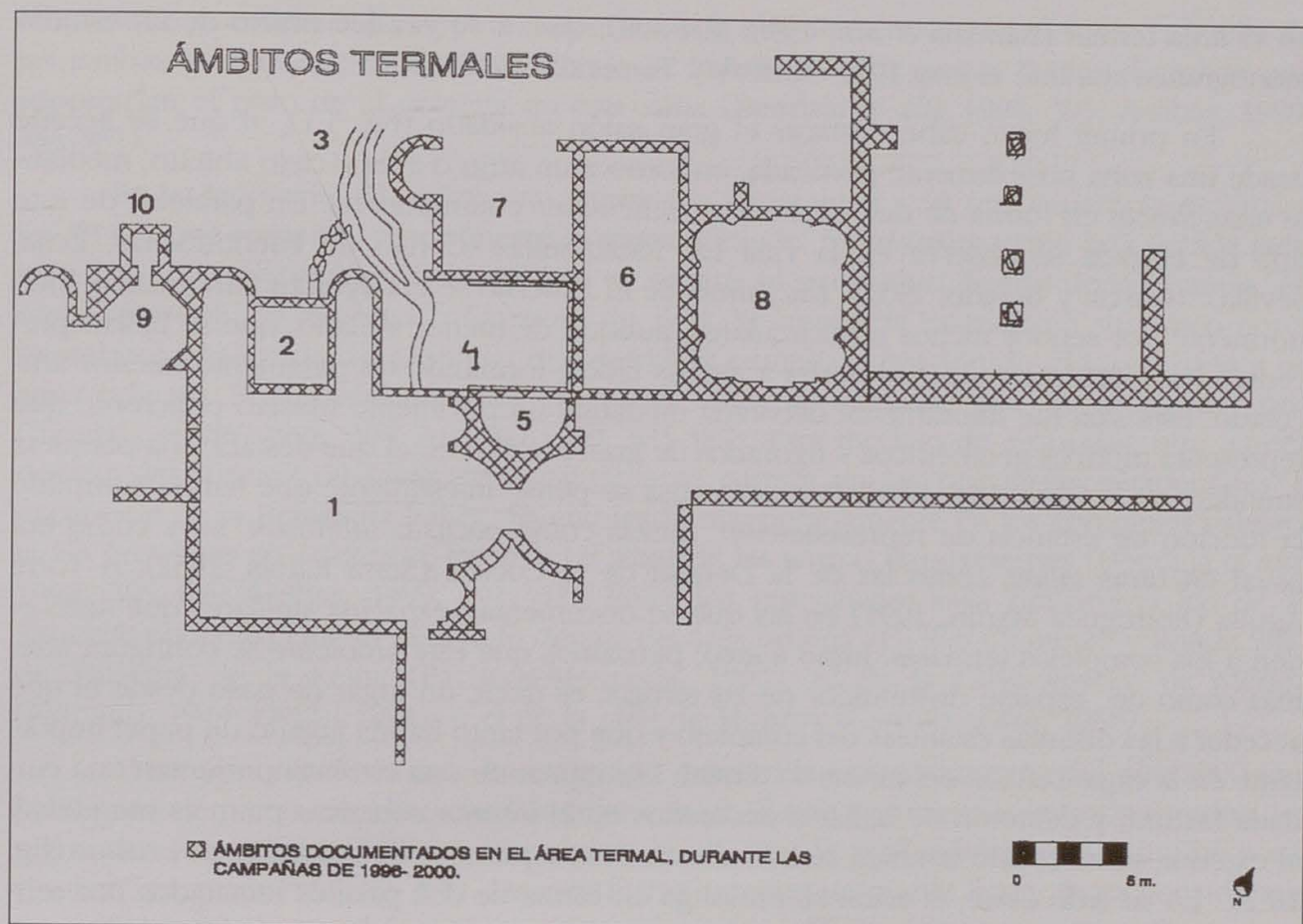
Figura 5. Planta del conjunto termal de El Saucedo .
