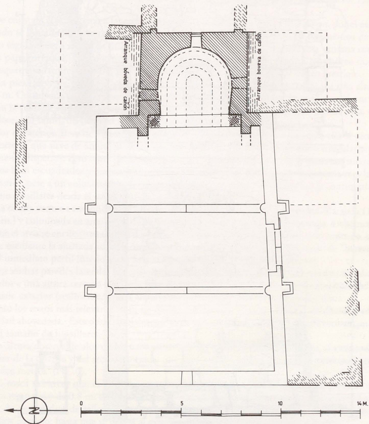
Fig. 4: Planta de la iglesia de San Miguel.
