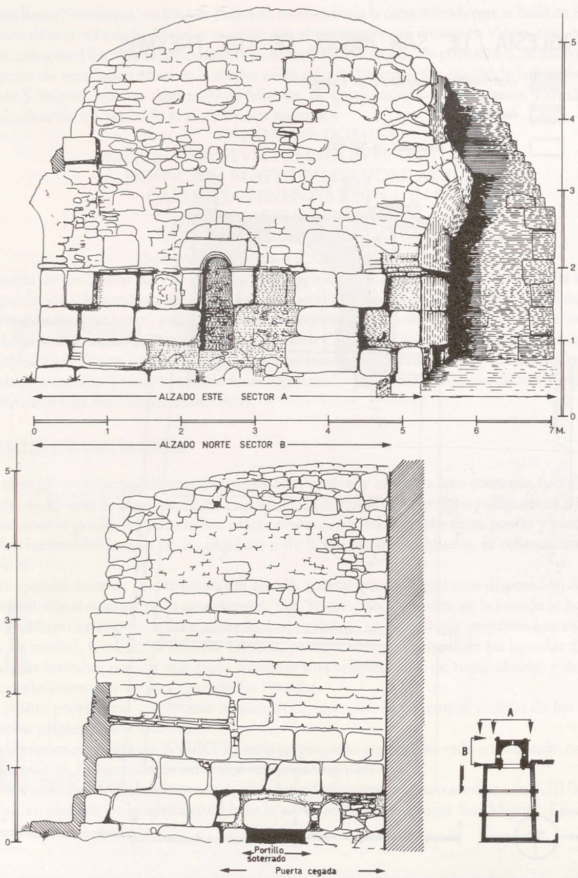
Fig. 5: Alzados Oriental y Septentrional del ábside central.
