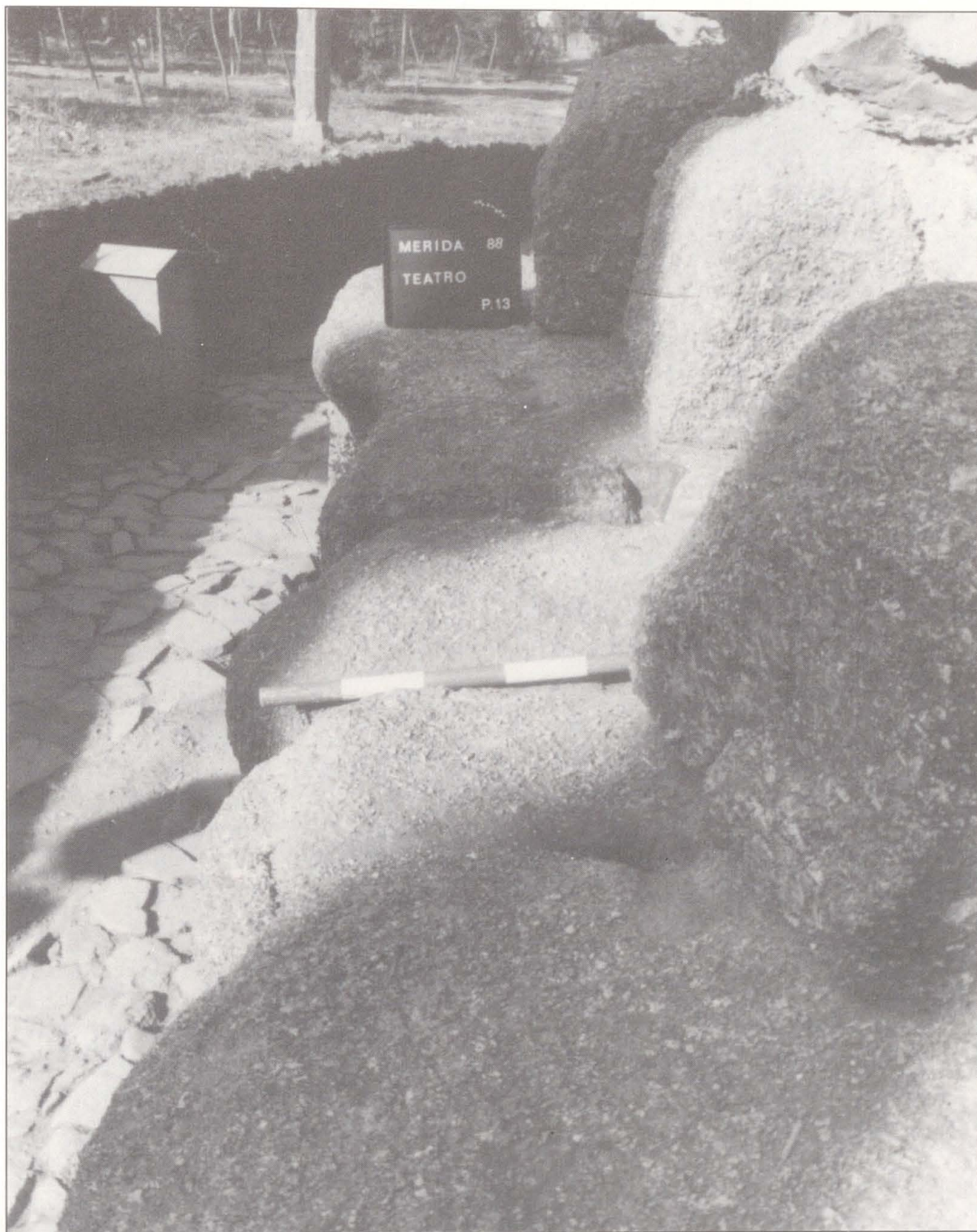
Lám. I) Detalle de la sucesión de mortajas ubicadas en las caras de recibimiento de los bloques y cómo cabalgan entre la línea de juntura. En primer plano, en la parte inferior aparece un orificio para los garfios. Nótese que se trata de una cara lateral del sillar.
