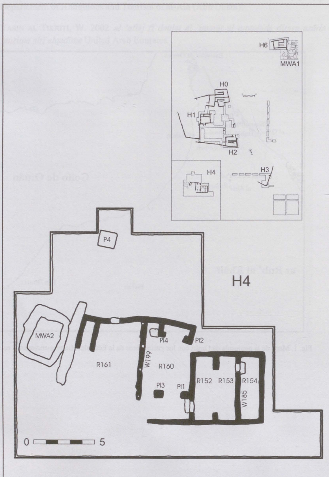
Fig. 2. Plano esquemático de AM1-Thuqaibah. (M.A. Núñez Villanueva, Misión española en al Madam).
