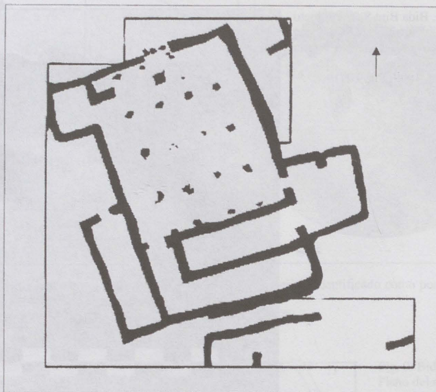
Fig. 12. Muweilah. Plano del edificio II del sector C, que muestra la sala de columnas. (Magee, plano cedido por el autor a la Misión española).
