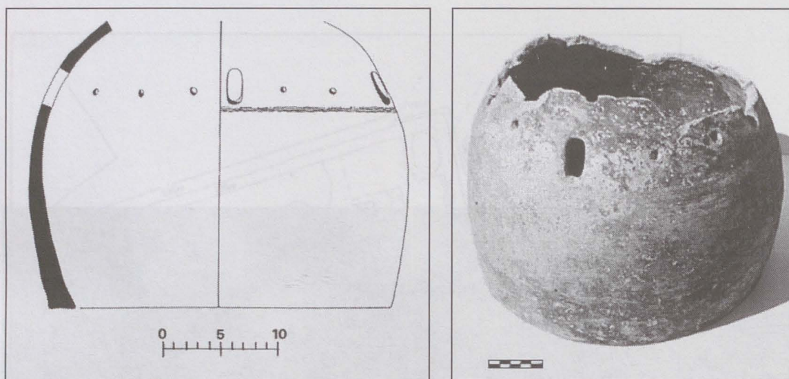
Fig. 8. Rumeilah. Objeto similar al incensario hallado en Muweilah, identificado como posible elemento utilizado en el sistema de distribución de agua de los aflaj. (Dibujo según Benoist 1999: Fig. 48.13; Foto según Benoist 1998).
