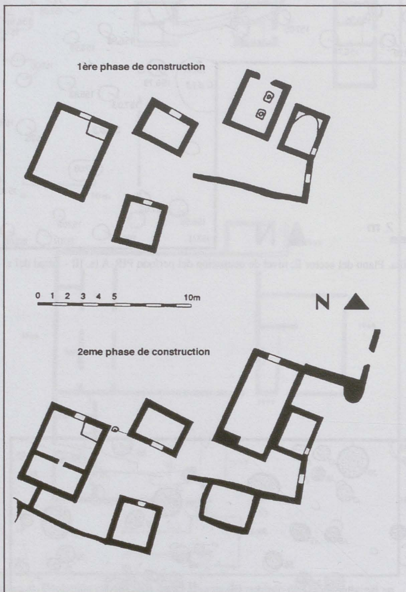
Figura 7. Mleiha. Plano esquemático mostrando la evolución de las casas excavadas en la zona este del sector L; período PIR-B (mitad del s. II - s. I a. C.)
