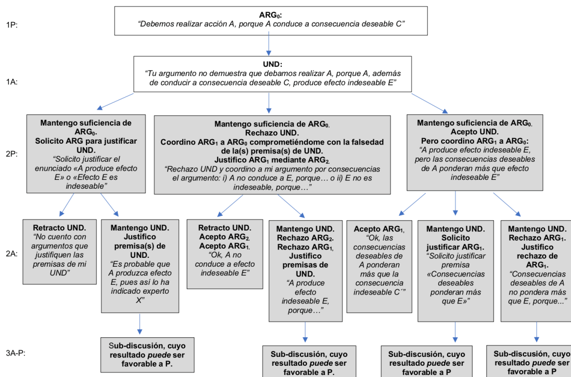
Fig. 5: Defensa exitosa de un argumento derrotable, frente a un undercutter (UND)
